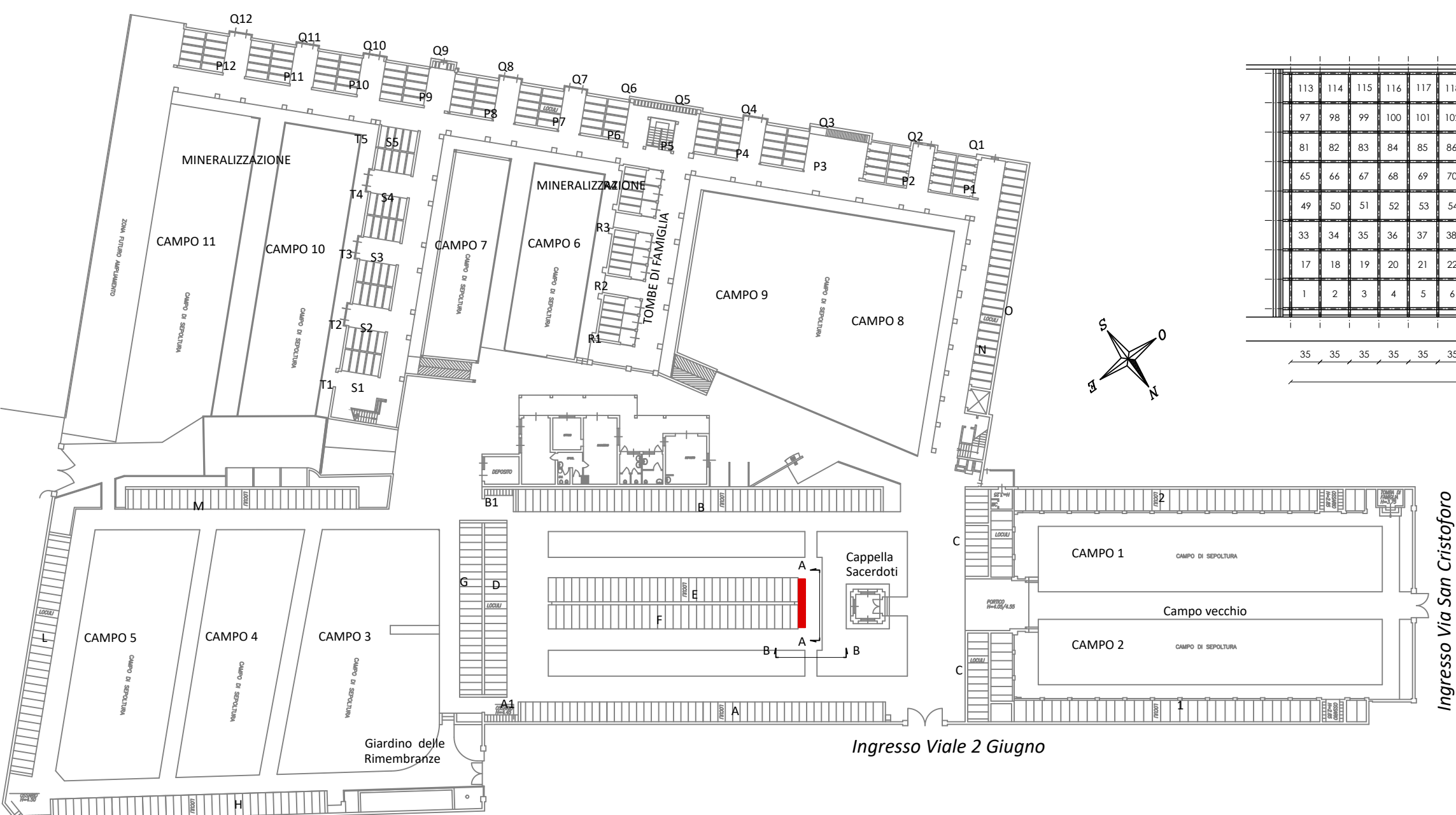
PLANIMETRIA GENERALE CON INDIVIDUAZIONE DELLE AREE OGGETTO DI INTERVENTO scala 1:1000
