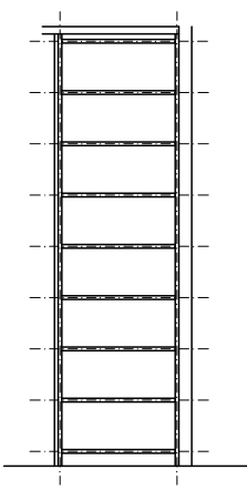
BATTERIA OSSARI SEZIONE B-B scala 1:50
